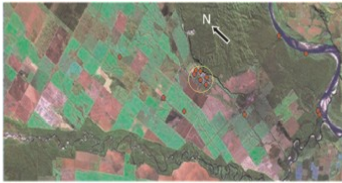
Figura 3 - Recorte de um cenário de NDVI, obtido de uma composição de imagens de satélite LANDSAT ETM. Observa-se o rio Bermejo (direita), Santa Maria (inferior) e Colorado (canto inferior direito). Os pontos vermelhos fora da circunferência amarela indicam os possíveis lugares de contatos rurais e os de dentro indicam os possíveis lugares de contatos urbanos nas zonas de Hipólito Yrigoyen. Dados: Hospital Eva Perón e Programa EDIS. Escala 1 cm: 1,5 km.
